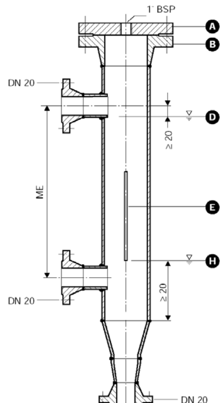
Rys.4 Zewnętrzne naczynie pomiarowe
